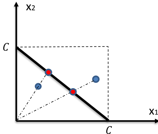
شکل (۷). مکان هندسی نقاط حل معادله
