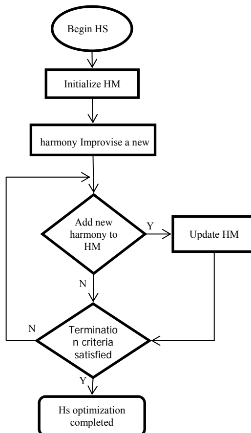
شکل ۵: فلوچارت الگوریتم جستجوی هماهنگی ساده
