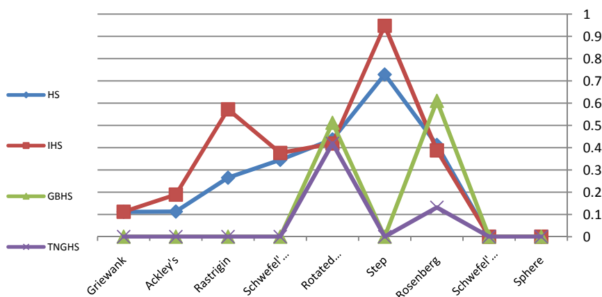
شکل ۱۴: نمودار مقایسه نتایج حاصل از حل هر مسئله در هر الگوریتم
