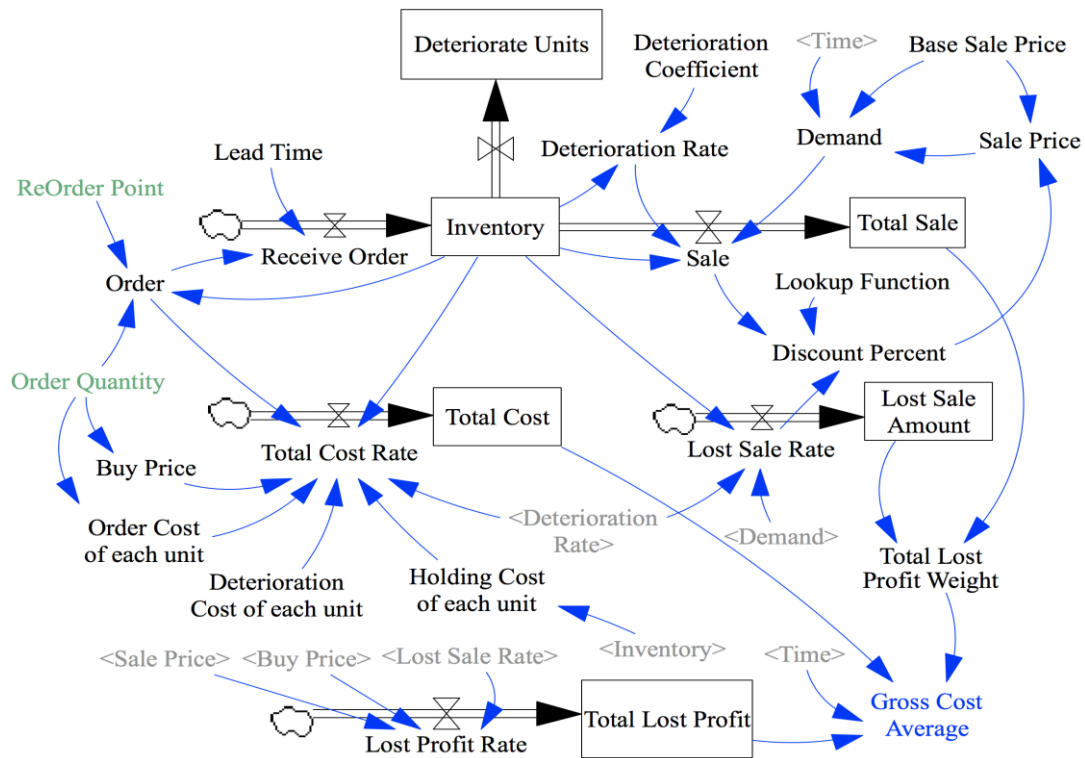
شکل (۸): نمودار جریان کنترل موجودی محصولات فسادپذیر در نرم‌افزار Vensim DSS
